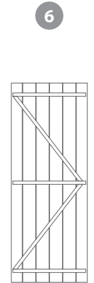
Door QTY 2 AI-R11FBMBZBD636X1660-V1
