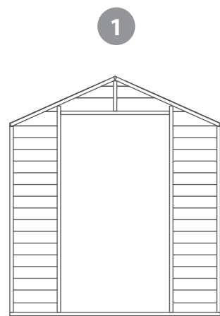
1 Door Gable QTY 1 AI-01R11OVAGSD1707X1961-V1
