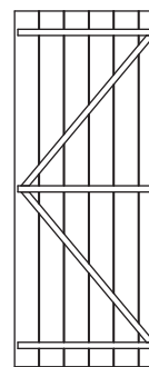
Door QTY 1 AI-R11FBMBZBD660X1600-V1
