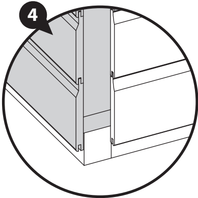
*External Corners*
